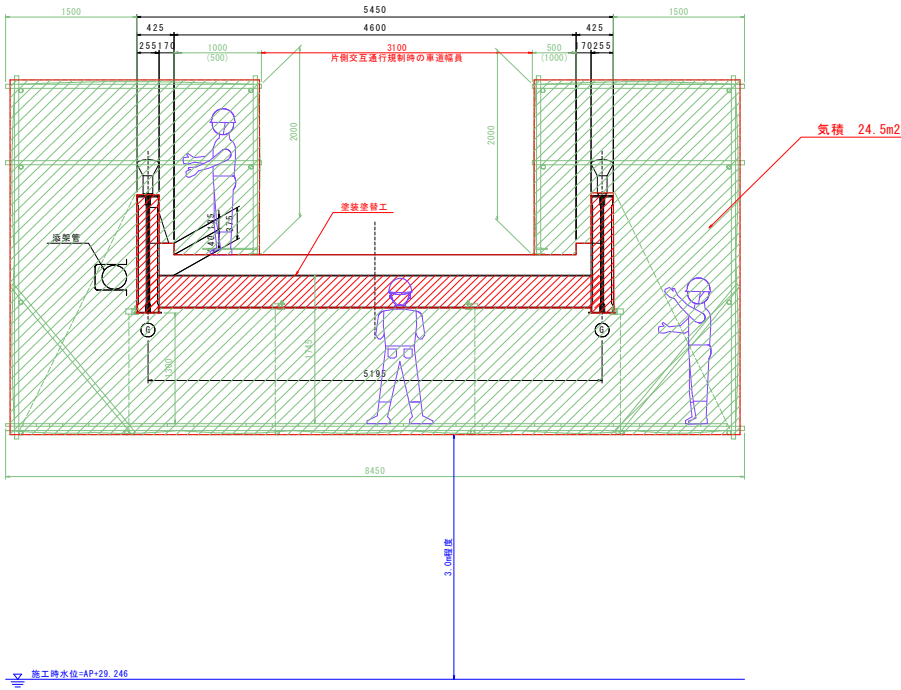
断面図 S=1:30
